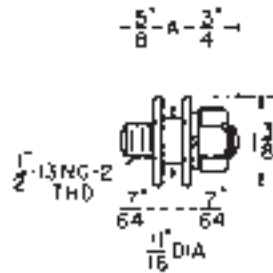
1/2" stud assembly
